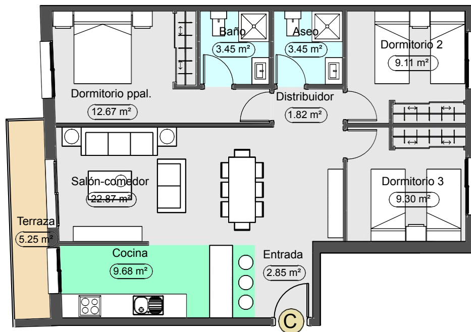
VIVIENDA C ESCALA 1:100
